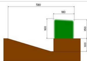
Nákres Velkého Taxisova příkopu
